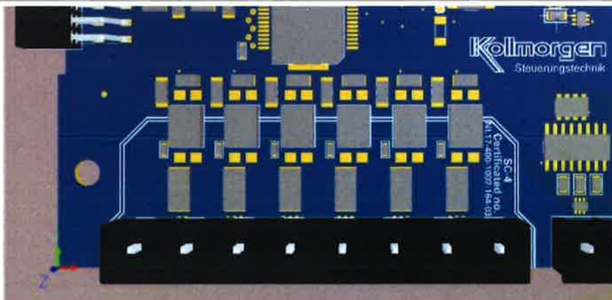
Impression neues Design mit Zertifikat-Nummer auf der SC-4 Schaltung gedruckt
